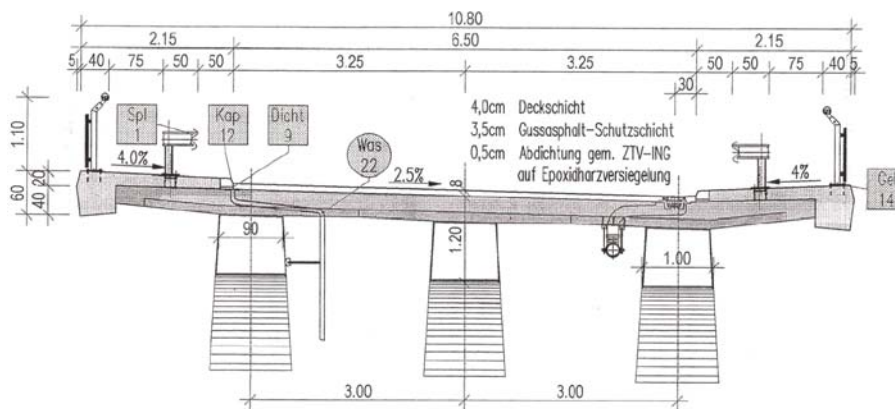
BW 47-1 Regelquerschnitt mit VFT-Träger
