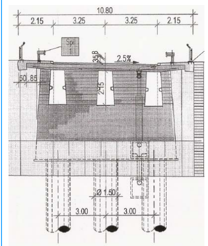
BW 47-1 Ansicht Rahmenstiel mit Bohrpfählfundung
